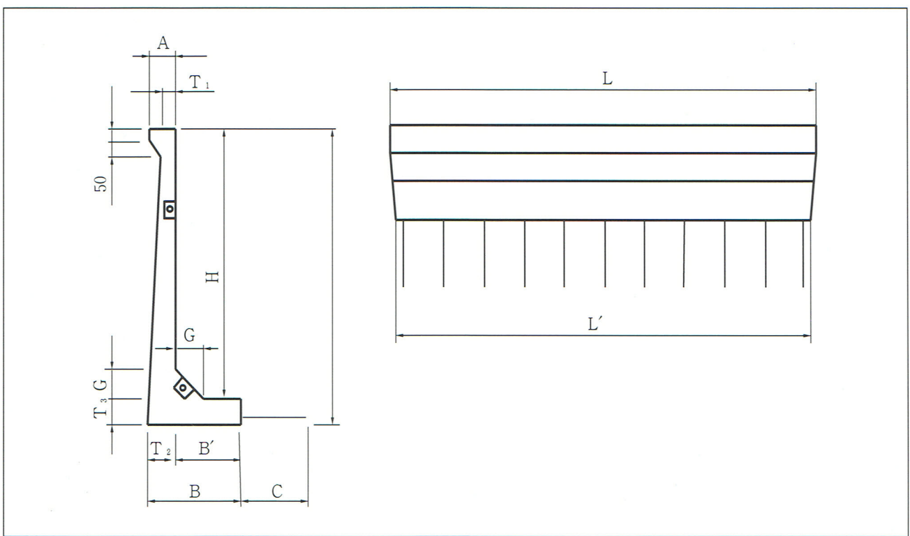
寸法表
