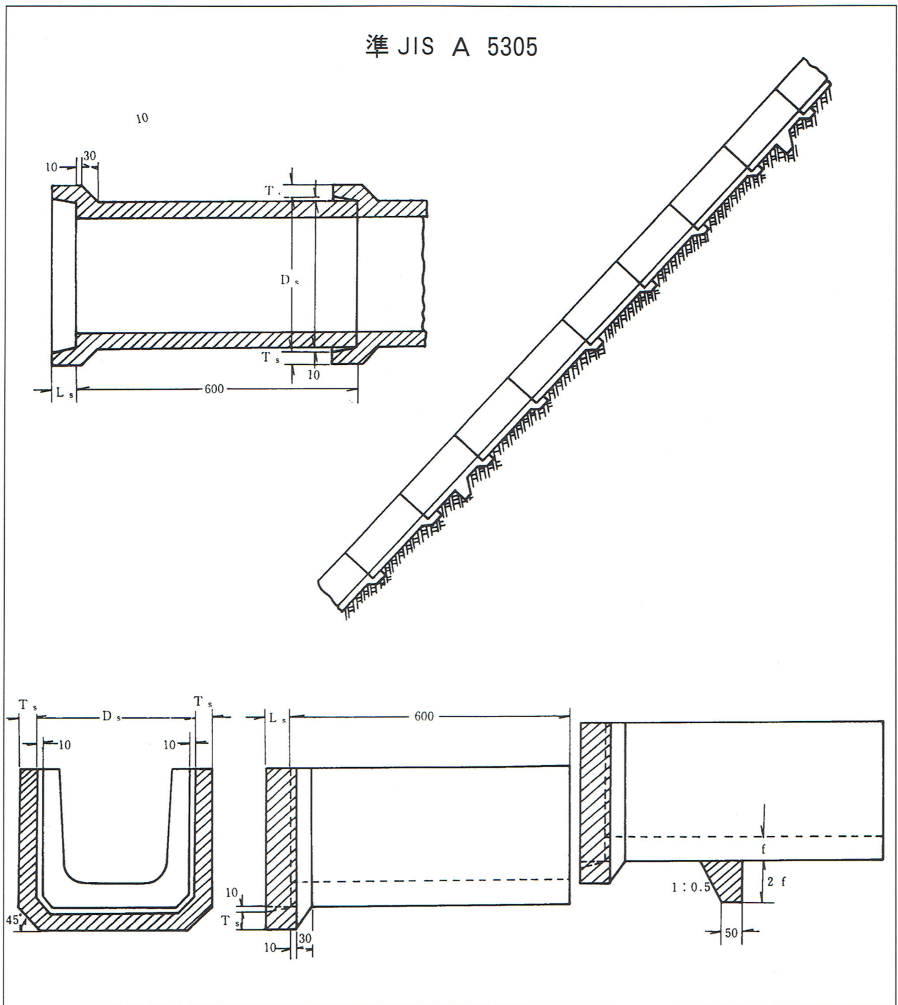
寸法・配筋表
